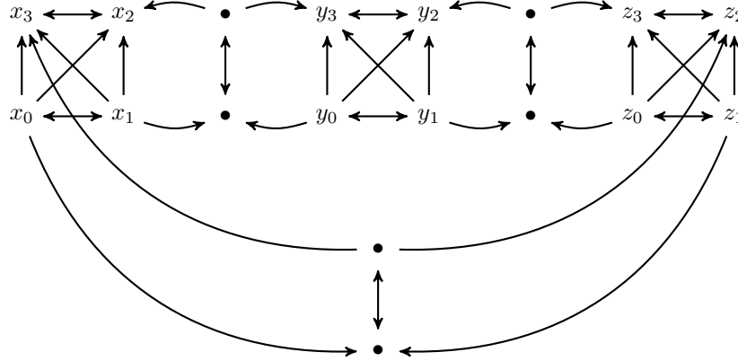
Fig. 6. Clause gadget
